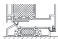
Hliníkový práh s přerušeným tepelným mostem do výšky 20 mm
