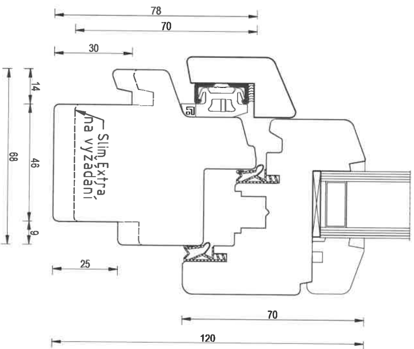
Alternativa typu: Rám dolní "Dřevěná okapnice"
