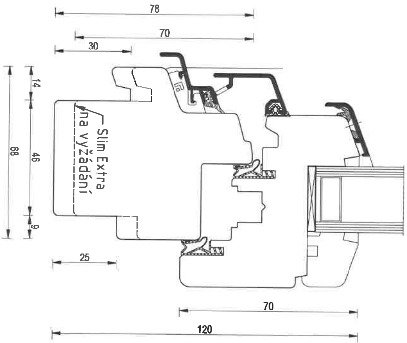
Alternativa typu: Rám dolní "Hliníková okapnice"
